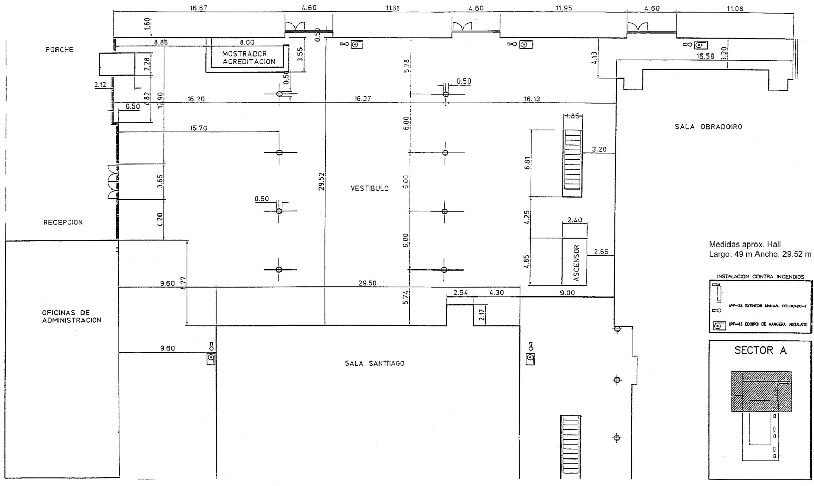
PLANTA SECTOR A
